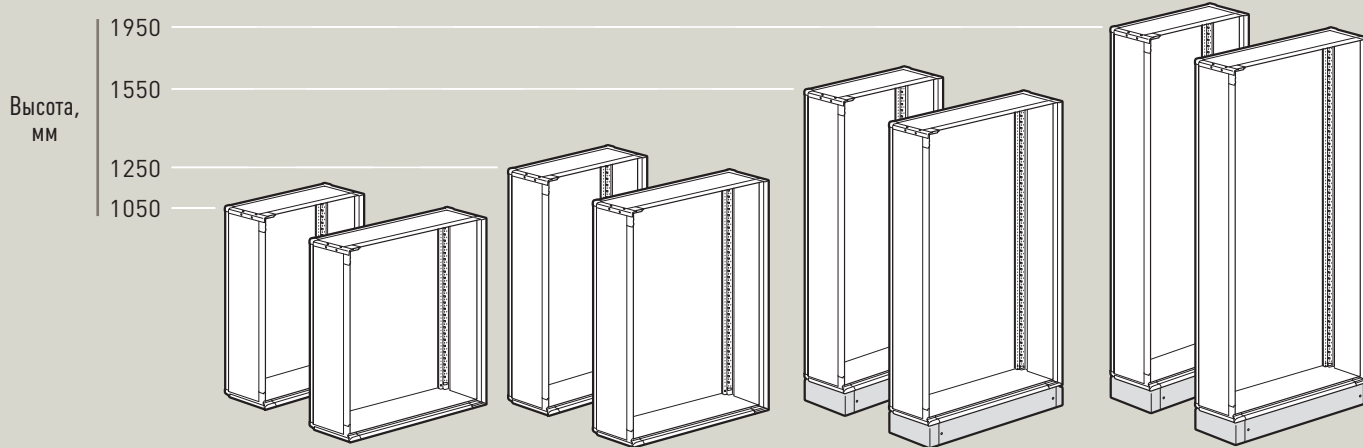
Распределительные щитки
